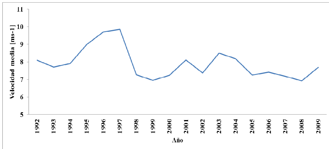
Figura 1. Velocidad media anual de viento a 10 m.
