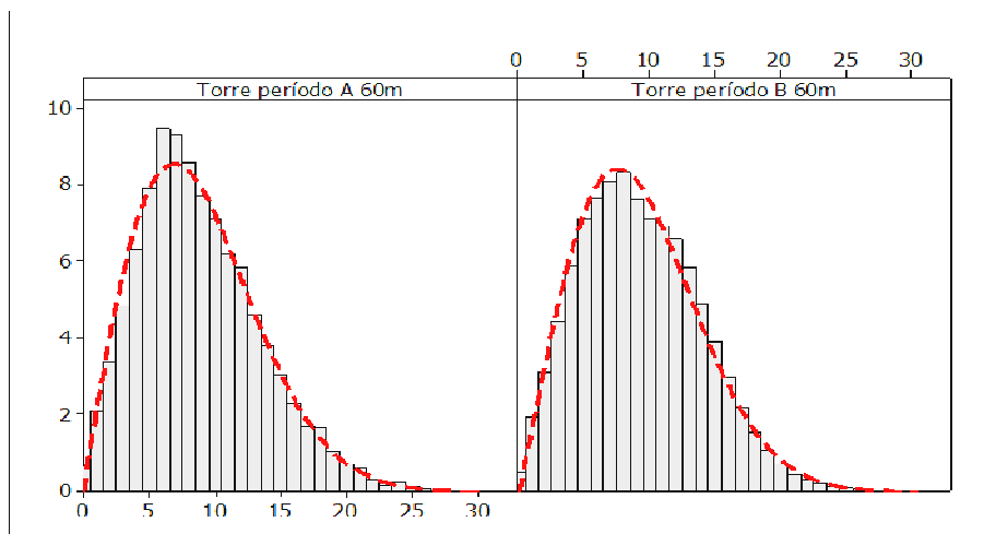
Figura 12. Distribución porcentual de velocidad para cada período de la torre (barras), ajustado con una distribución teórica de Weibull (línea punteada roja). Los valores del eje x son en \text{ms}^{-1} .
