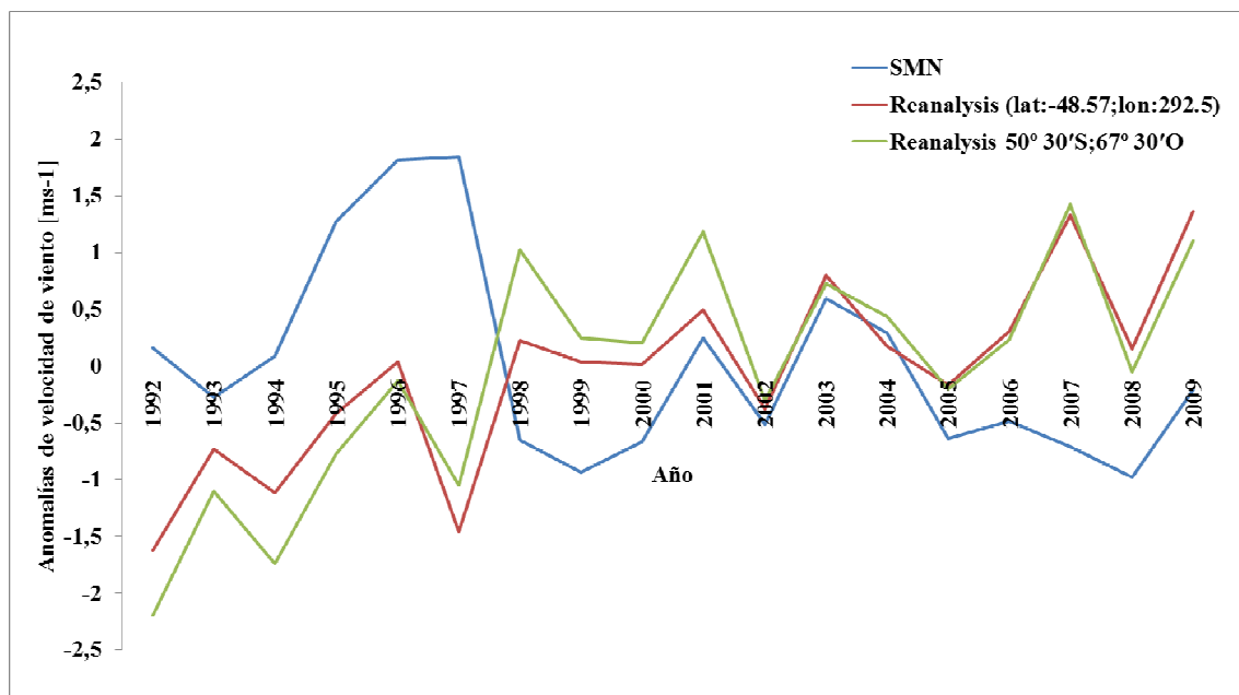
Figura 2. Anomalías anuales de velocidad del viento para San Julián Aero (línea azul) y dos puntos de la base de datos de R2 (línea roja punto sobre tierra y línea verde punto sobre el mar).
