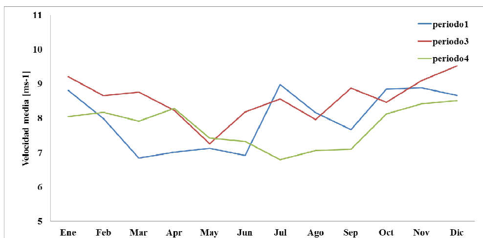
Figura 6. Ciclo anual de velocidad de cada período.
