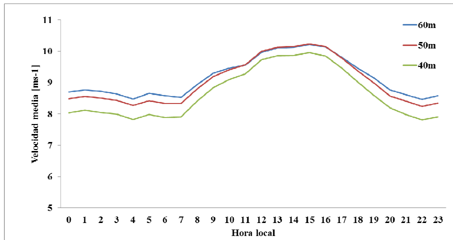
Figura 13. Ciclo diario de velocidad para cada altura en la torre del período B. Los valores de velocidad son promedio de ambos canales de medición a excepción del canal de 40 m.
