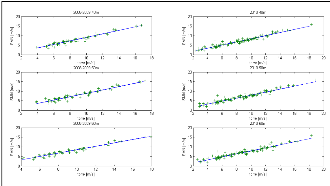
Figura 14. Diagramas de dispersión entre el vientos medio diario a 10 m y a 40 m, 50 m y 60 m para períodos coincidentes. Período 2008-2009 (A) Período 2009-2010 (B).
